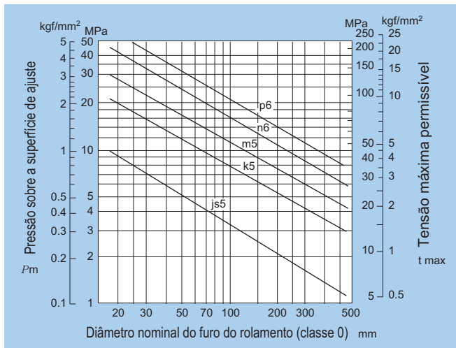
Fig.17.5.1 Interferência média de ajuste em relação à pressão da superfície ( P_m ) e à tensão máxima permissível ( t_{max} )
