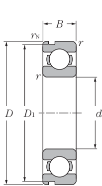
Com ranhura para anel elástico
