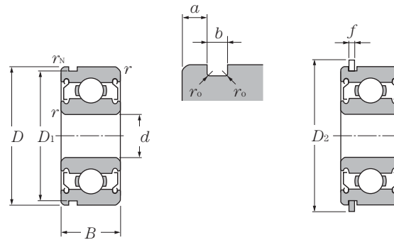
Ranhura para anel elástico Tipo blindado (ZZ)
