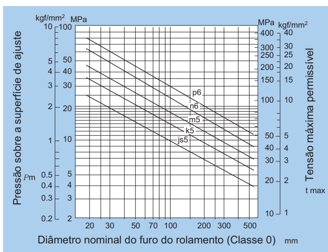
Fig.17.5.2 Interferência máxima de ajuste em relação à pressão da superfície ( P_m ) e à tensão máxima permissível ( t_{max} )
