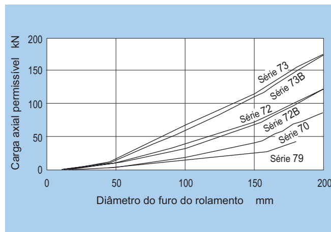
Fig. 17.4.2 Carga axial permitível para rolamentos de esferas de contato angular
