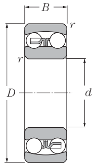
Furo cilíndrico
