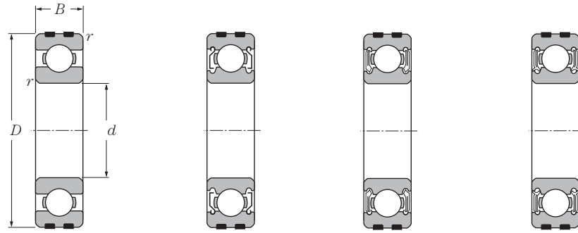
Aberto
