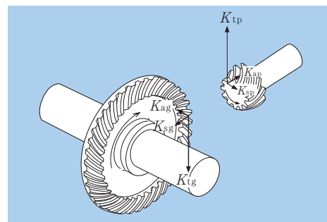
Fig. 4.4 Cargas sobre engrenagens cônicas
