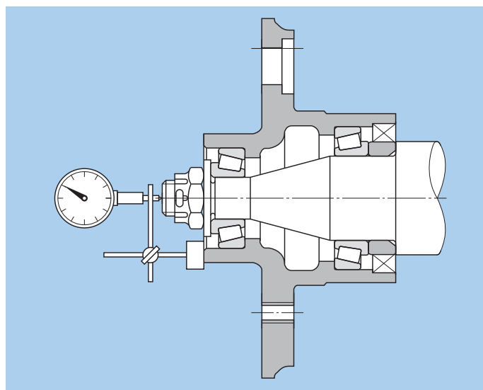
Fig. 15.13 Medição do ajuste da folga interna axial
