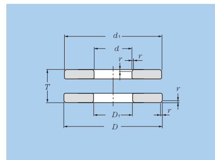
Fig. 5.3 Rolamentos axiais de escora simples
