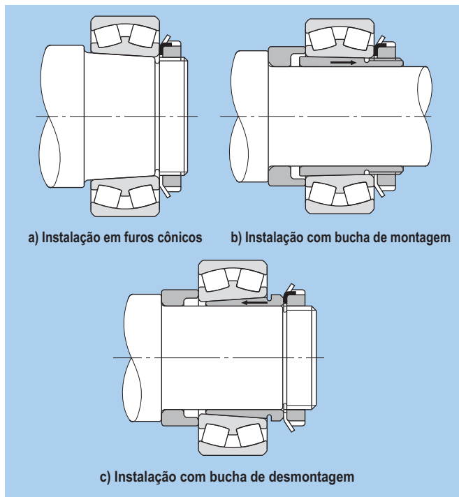
Fig. 15.7 Métodos de instalação utilizando porcas de fixação
