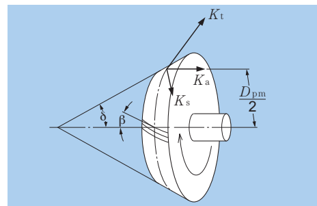
Fig. 4.5 Diagramas de engrenagens cônicas
