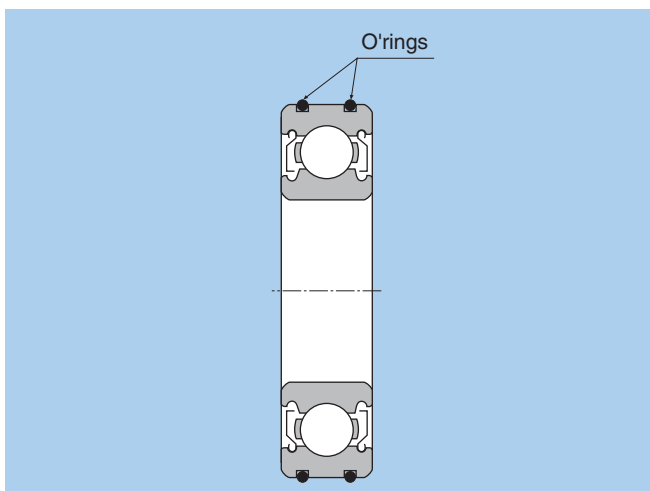
Fig. 3. Rolamento AC
