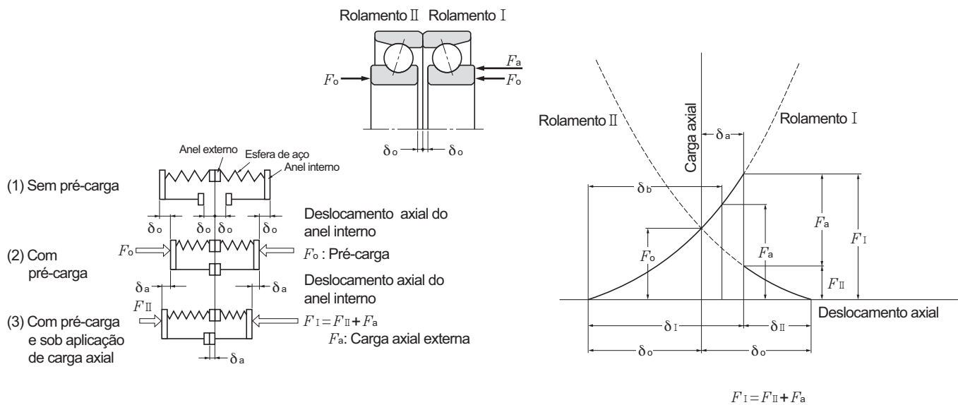
Fig. 8.2 Pré-carga por posição fixa e deslocamento axial
