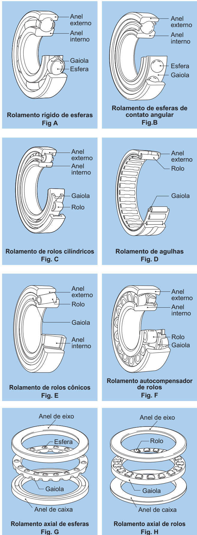
Fig. 1.1 Rolamentos
