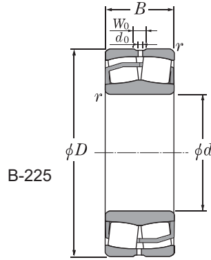
Furo cônico tipo EA
