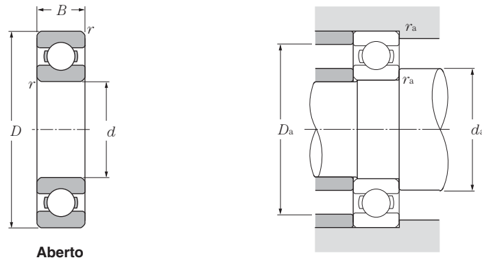
Aberto
