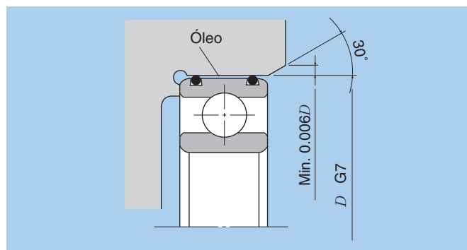
Fig. 4. Alojamento
