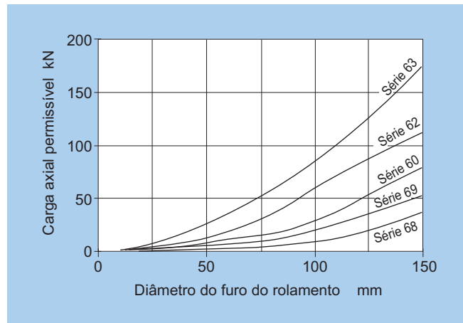
Fig. 17.4.1 Carga axial permitível para rolamentos rígidos de esferas
