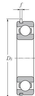
Com anel elástico
